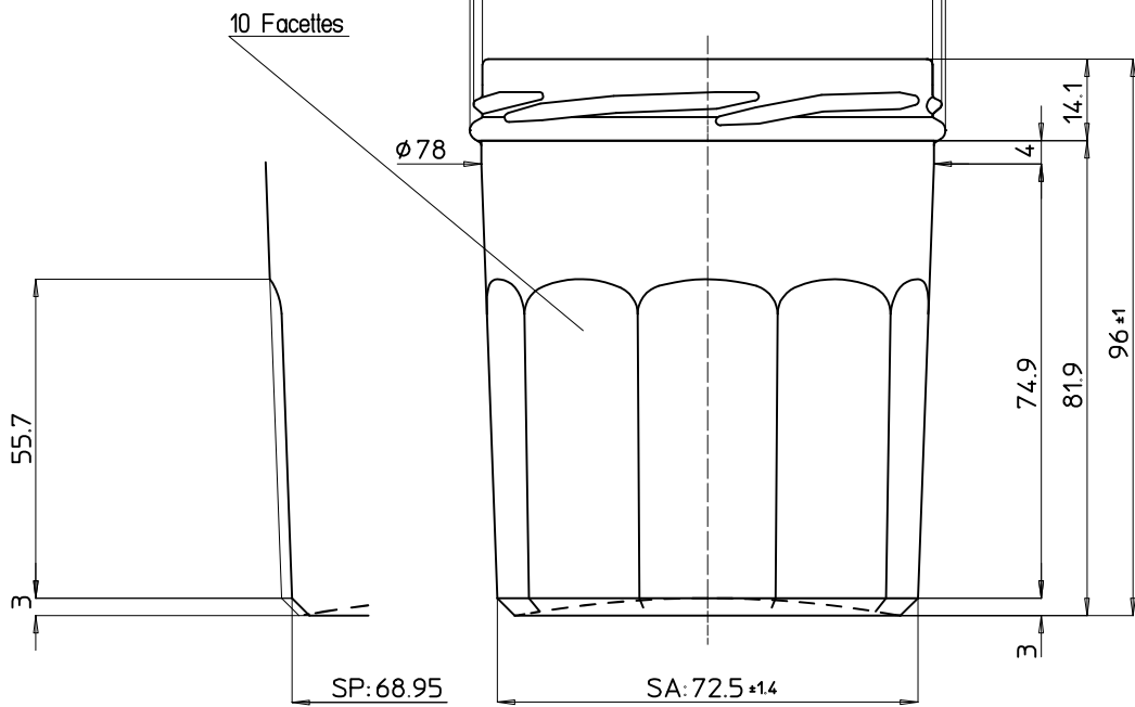
Coupe partielle suivant A A
